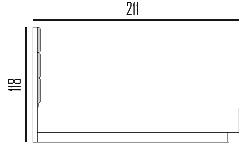
YAN GÖRÜNÜS SIDE VIEW
