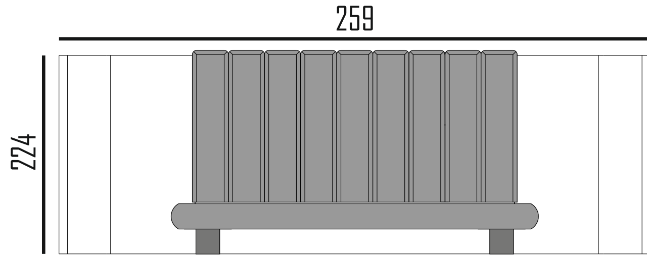
ÖN GÖRÜNÜS FRONT WIEW
