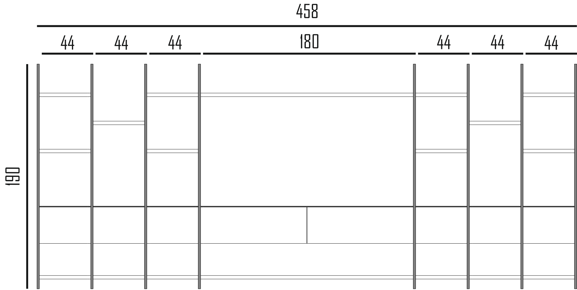
ÖN GÖRÜNÜS FRONT VIEW
