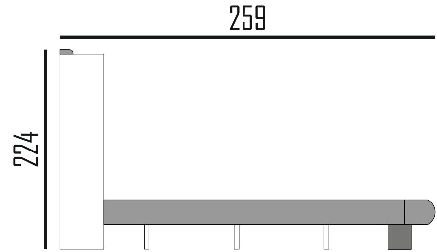
YAN GÖRÜNÜS SIDE WIEW
