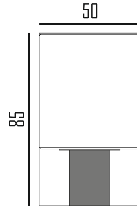
YAN GÖRÜNÜS SIDE VIEW
