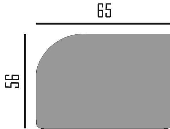
ÜST GÖRÜNÜS TOP VIEW
