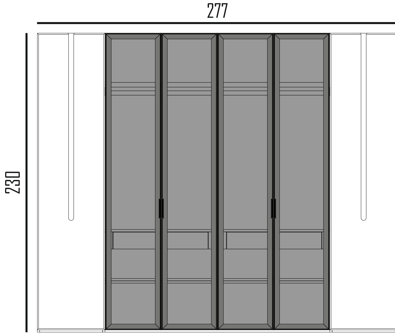
ÖN GÖRÜNÜS FRONT VIEW
