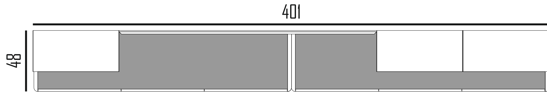
ÜST GÖRÜNÜS TOP VIEW
